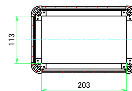
C-C ( 1 : 5.5 )
