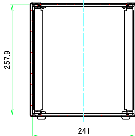
A-A ( 1 : 5.5 )
