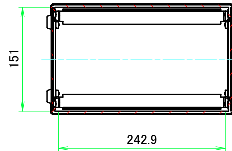
B-B ( 1 : 5.5 )
